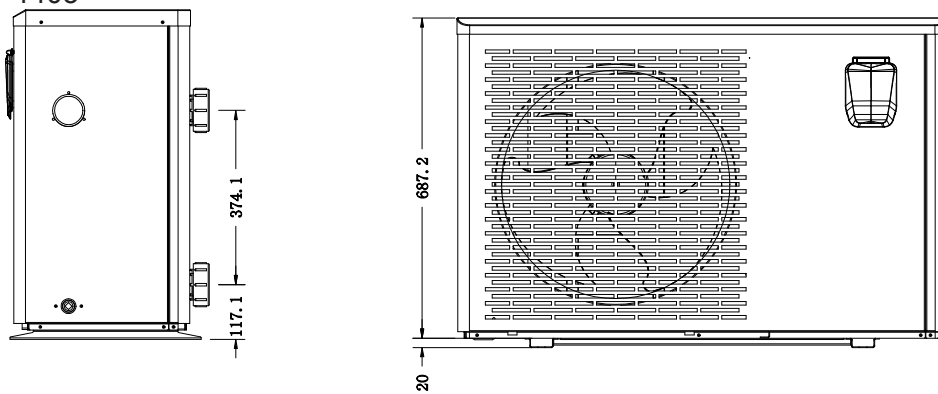
Wärmepumpe 1402 und 1403
