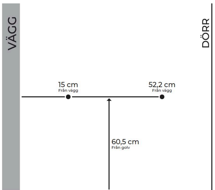
Ritning på montering av skruvar
