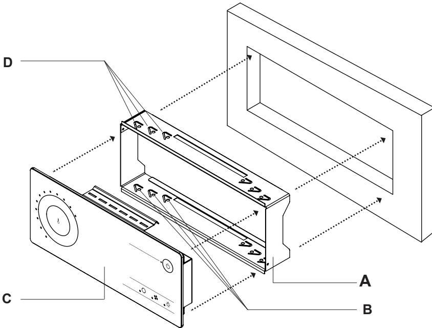
Kuva 3 Hallintalaitteen asentaminen
