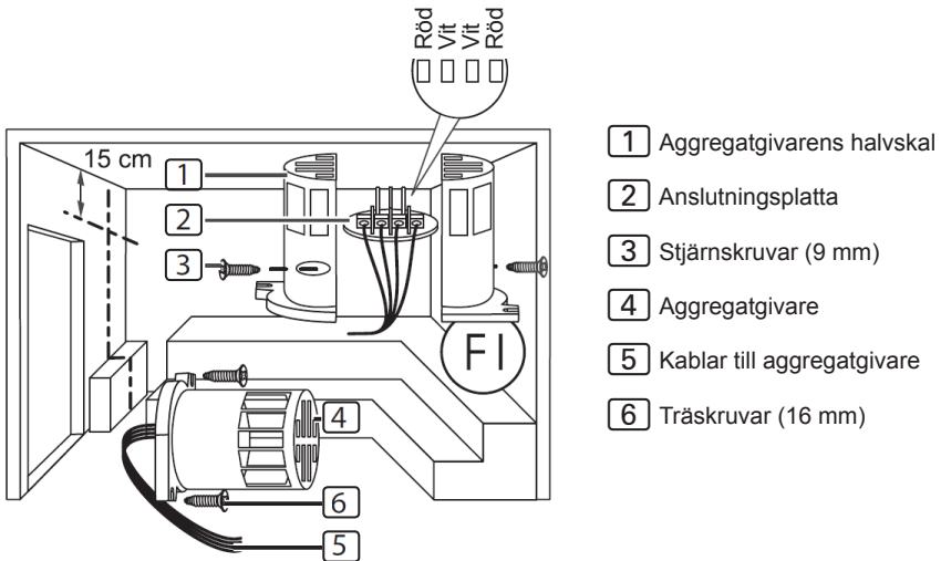
Bild 4 Montera aggregatgivaren (F1)
