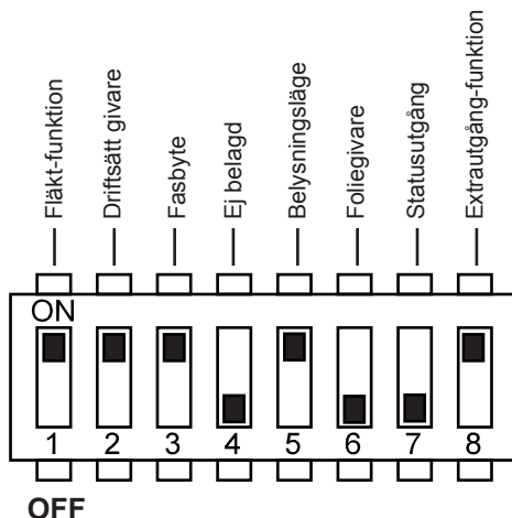
Bild 6 Funktionsomkopplare - standardinställning
