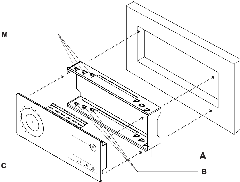
Bild 3 Montering av manöverreglaget
