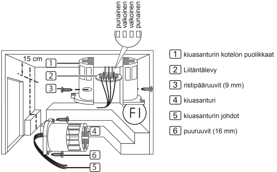
Kuva 4 Kiuasanturin (F1) asentaminen
