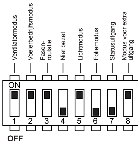
afb. 6 Functiekeuzeschakelaar – standaardinstelling
