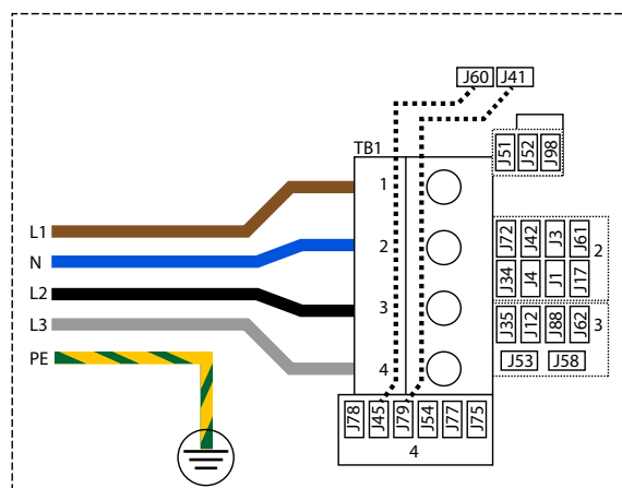
400v 16A Anslutningsdiagram Swimdelen.
