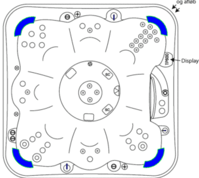
Udespa Riptide, 216 x 216 x 97 cm. Hjørneradius 30cm
